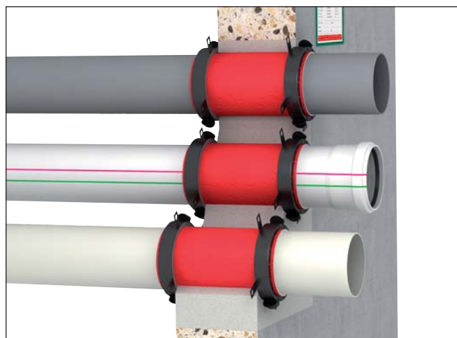
Passage paroi avec isolant
