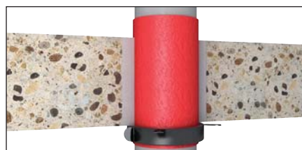
Installation sur plafond \geq 150 mm avec feuille insonorisante en PE.
