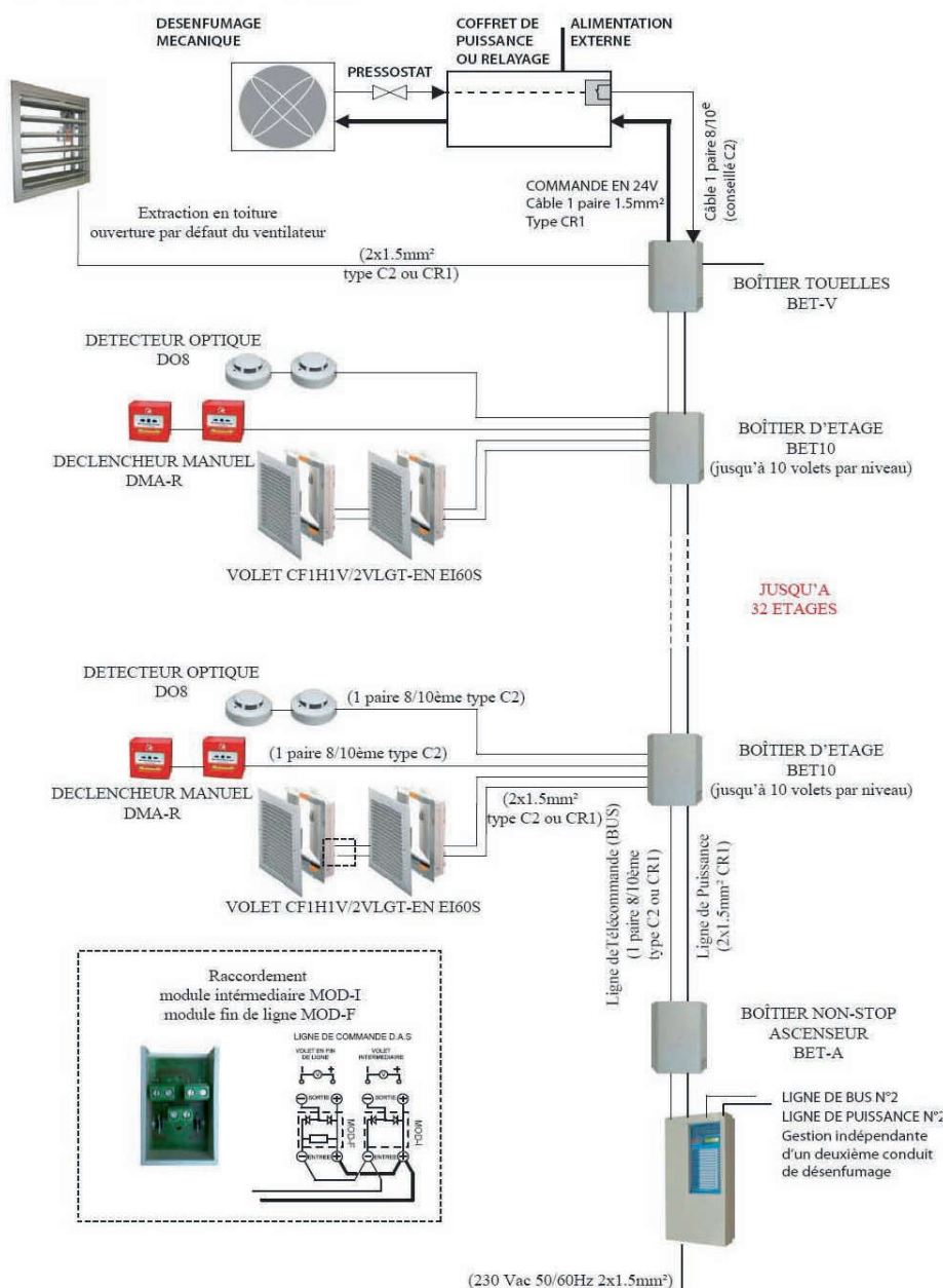
Modules MOD-I et MOD-F
